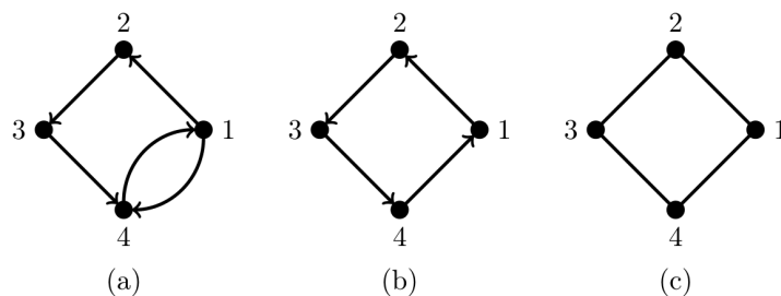
Figura 2: (a) Un digrafo que no es grafo orientado porque tanto 1 \rightarrow 4 como 4 \rightarrow 1 son aristas; (b) un grafo orientado que se puede obtener dando orientaciones a las aristas del grafo (c).
