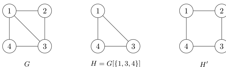
Figura 3: Un grafo G y dos subgrafos H y H' . El subgrafo H es inducido, mientras que el subgrafo H' no lo es, porque le falta la arista (1, 3) .
